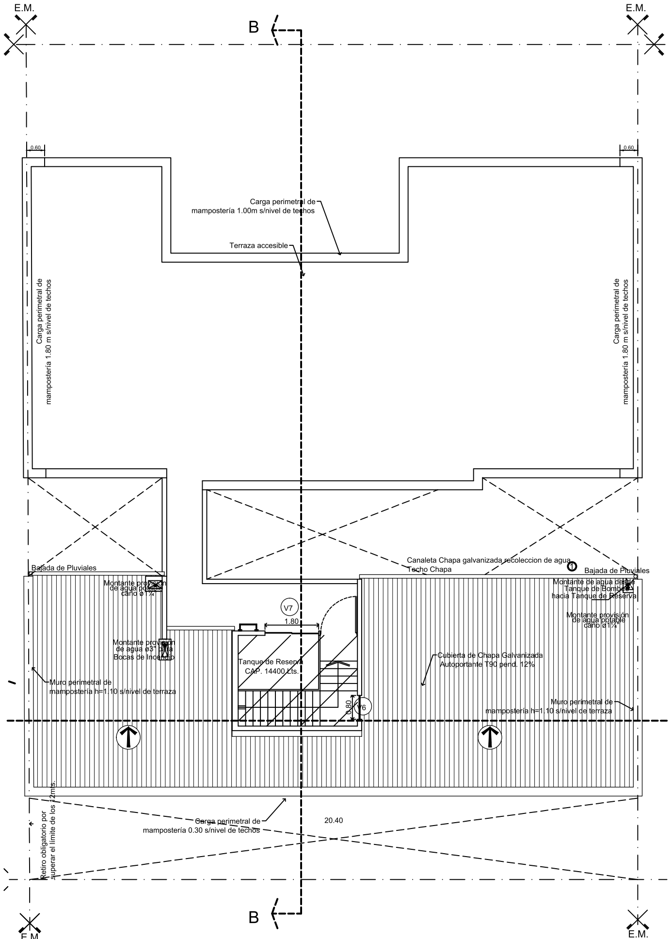
PLANTA DE TECHOS TERRAZA - CULLEN 862 - ESPERANZA
